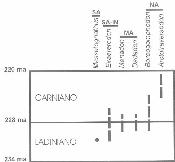
Figura 5. Cinodontes traversodontidos que presentan rasgos morfológicos compartidos con las nuevas formas de Santa Cruz do Sul. IN: India; MA: Madagascar; NA: Norteamérica; SA: Sudamérica. Escala temporal según Ross et al. (1994).
