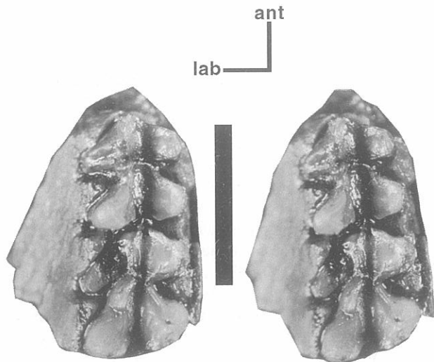
Figura 4. Traversodontid Tipo III. Estereopar del fragmento del maxilar con cuatro postcaninos (MCN PV 2748) en vista ventral. Escala 5 mm. Traversodontid Type III. Stereo pair of maxillary fragment with four postcanines (MCN PV 2748) in ventral view. Scale 5 mm.
